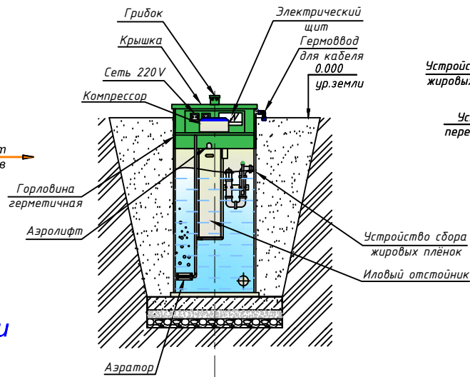
Разрез В-В
