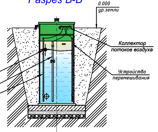
Разрез Б-Б
